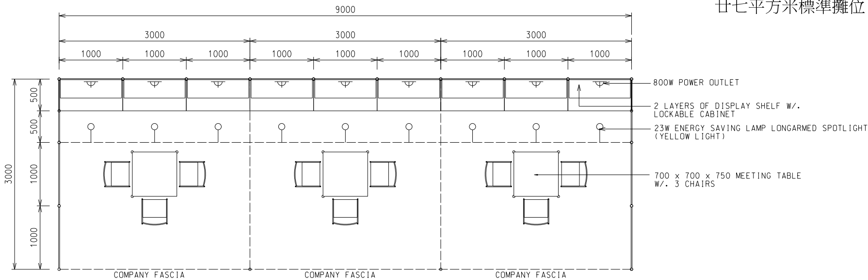
PLAN 9M(W) X 3M(D) X 2.5M(H) Standard Booth A
